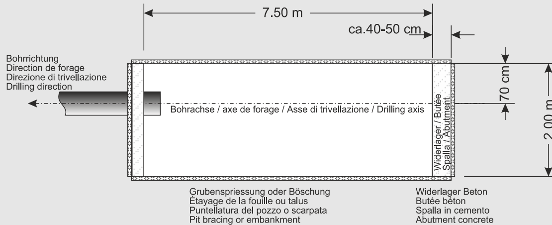
Grundriss / Coupe horizontale / Proiezione orizzontale / Top view
