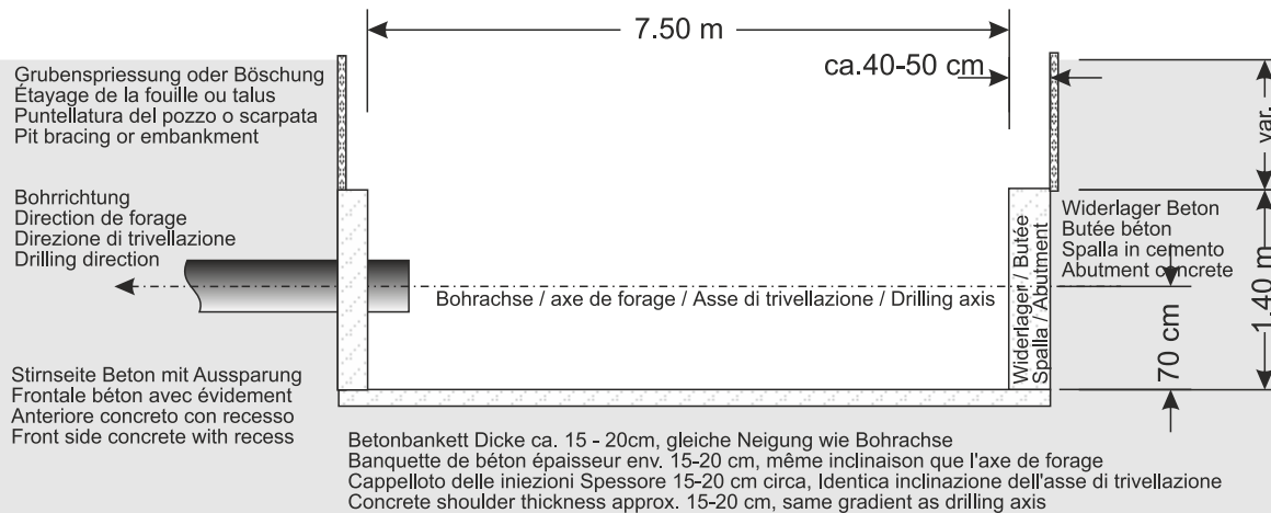
Schnitt / Coupe verticale / Proiezione verticale / Side view
