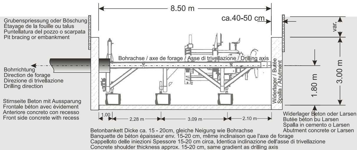
Schnitt / Coupe verticale / Proiezione verticale / Side view
